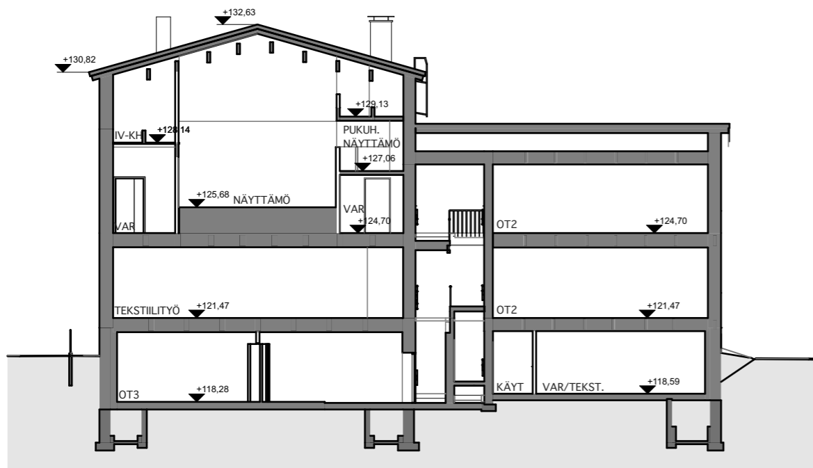
Leikkaus B-B
