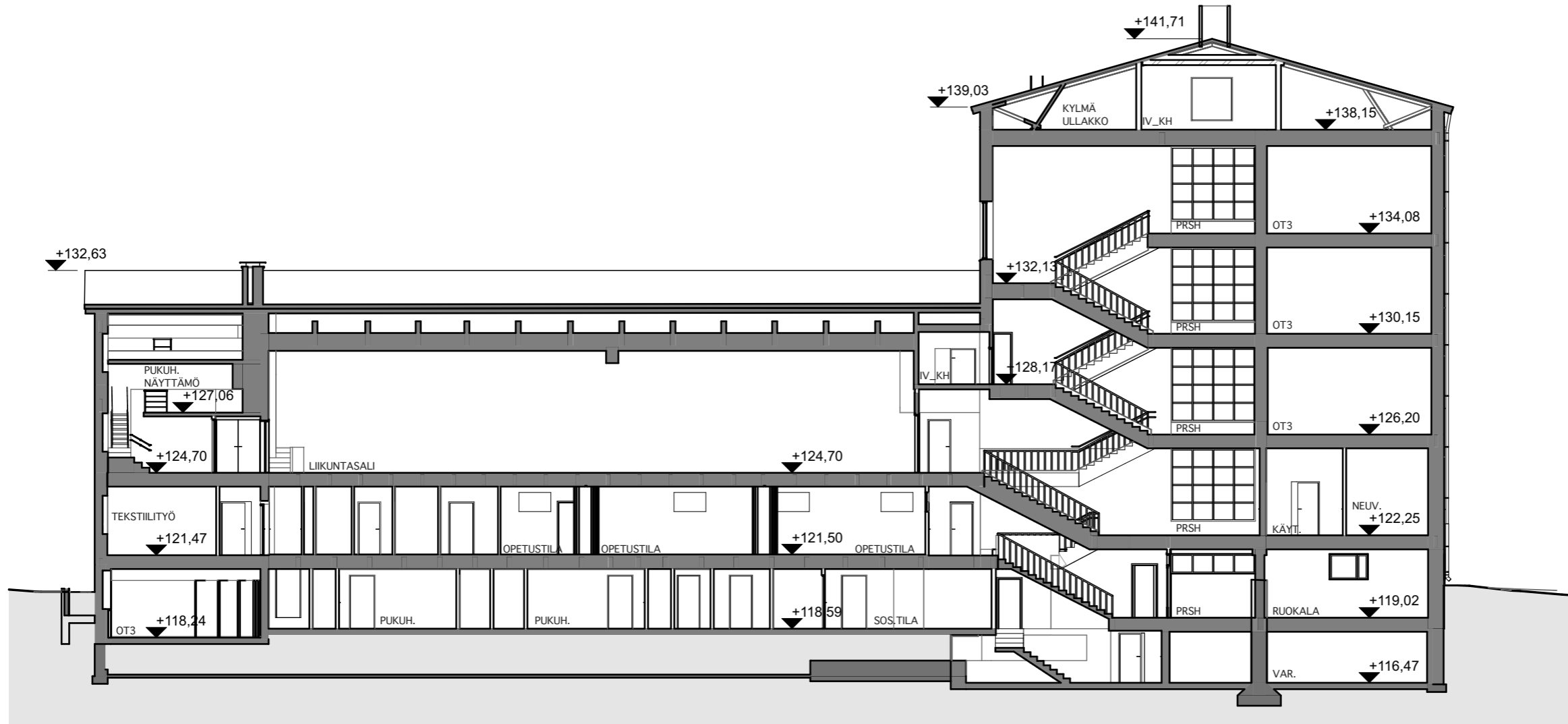
Leikkaus A-A
